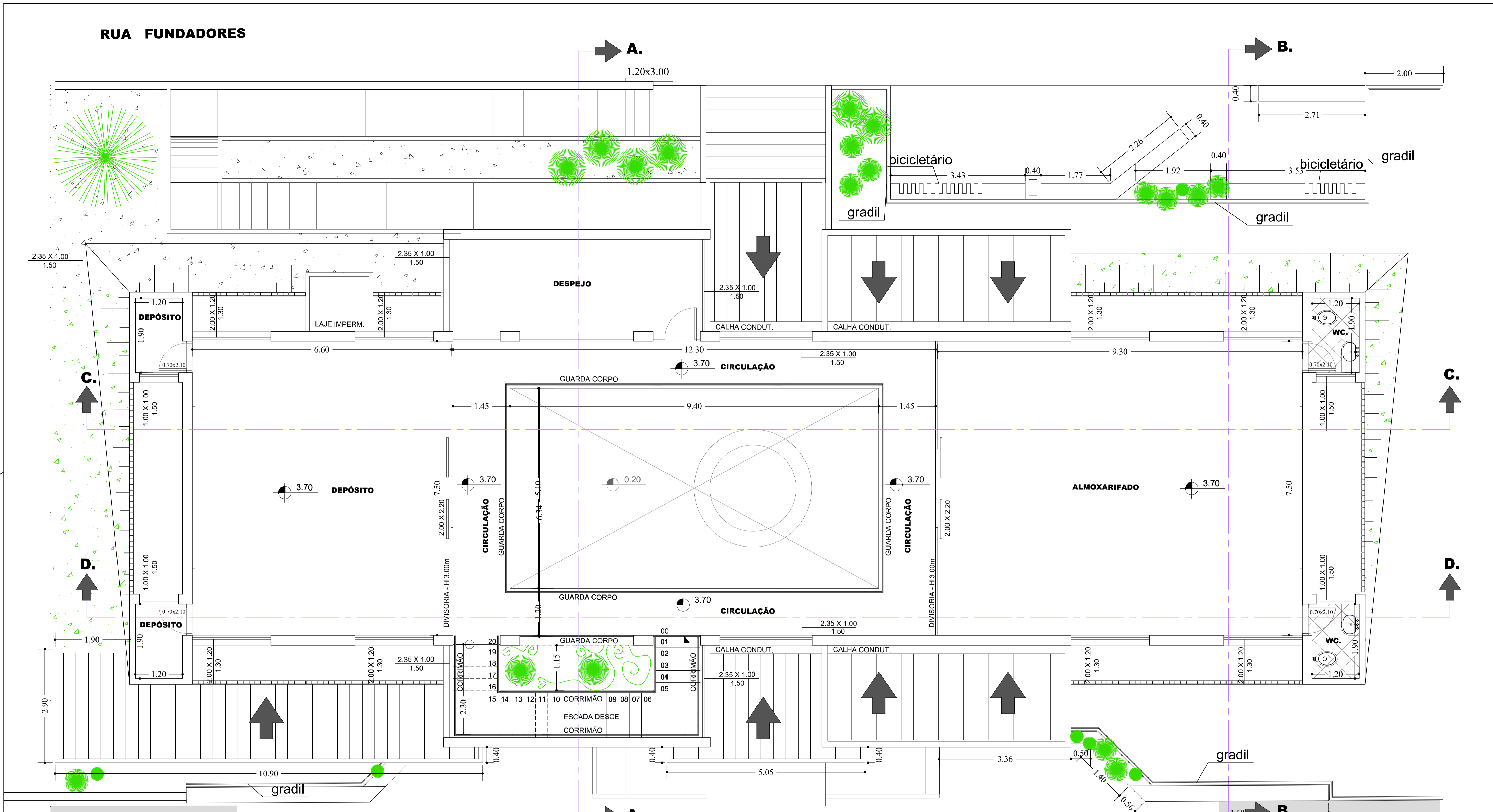
PROJETO DE ARQUITETURA (PAVIMENTO SUPERIOR) ESCALA GRAFICA: (1:50)
